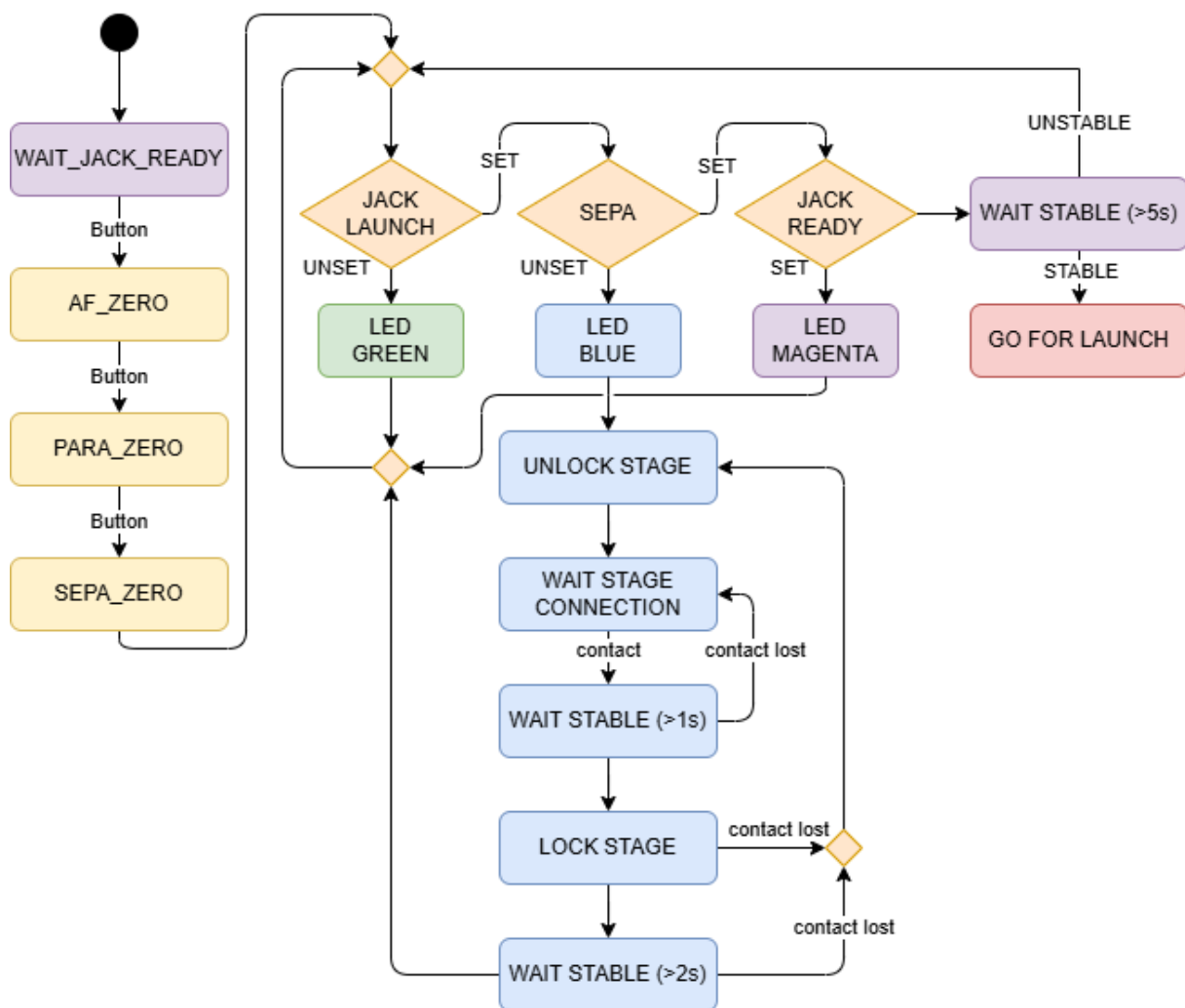
FIGURE 1.10 – Phase d'initialisation du premier étage.
