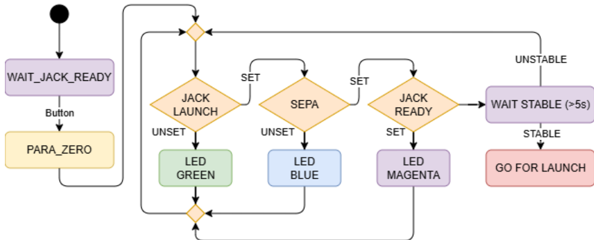
FIGURE 1.12 – Phase d'initialisation du deuxième étage.
