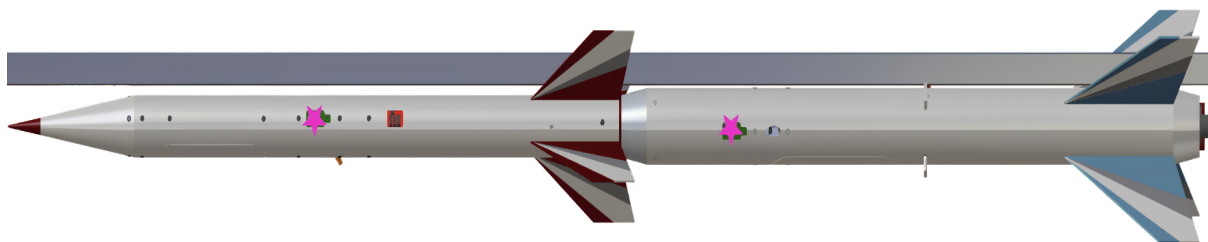
FIGURE 1.17 – Etages assemblés en rampe, indicateur magenta sur les deux étages.
