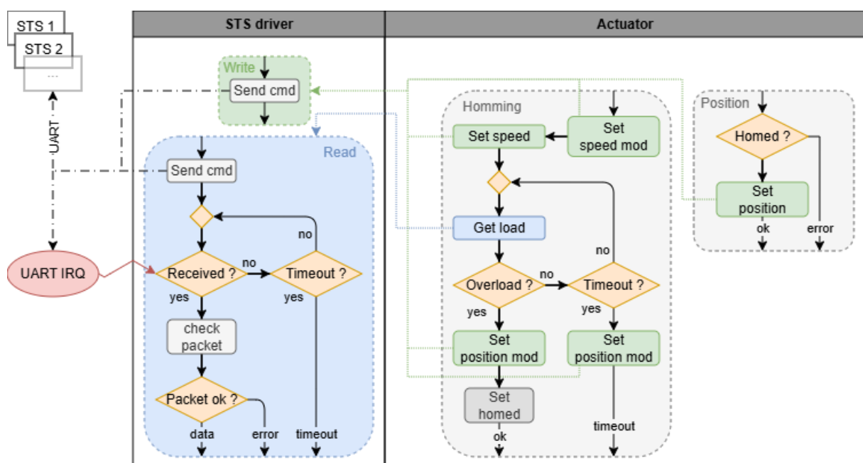
FIGURE 1.23 – Articulation du pilote STS et de l'utilitaire actuator
